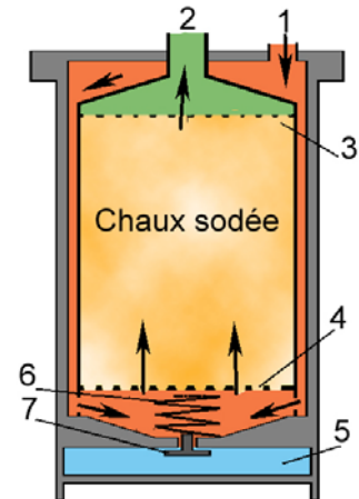
Scrubber moulé – Dräger
