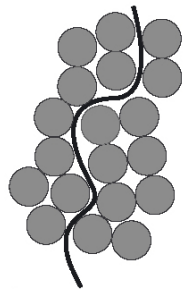
Granule sphérique
